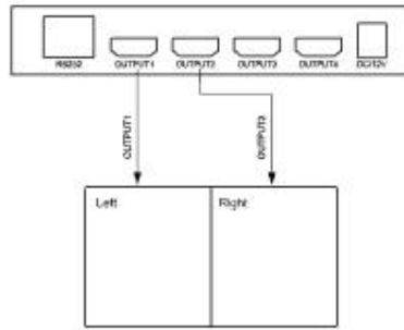
Left---OUTPUT1/OUTPUT3 Right---OUTPUT2/OUTPUT4
